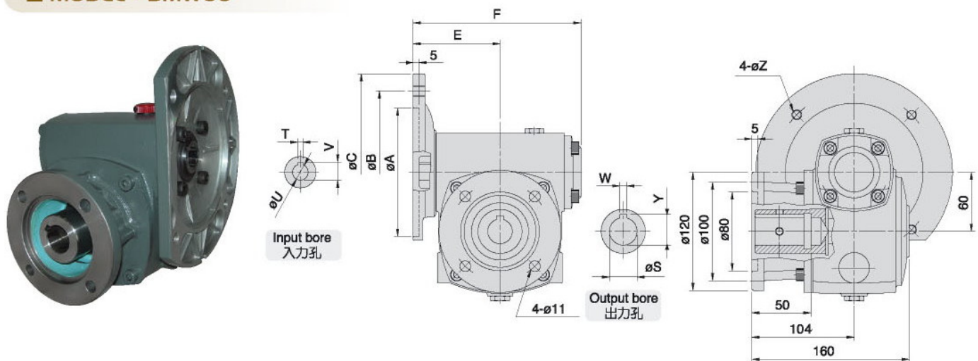
尺寸表 Dimension
