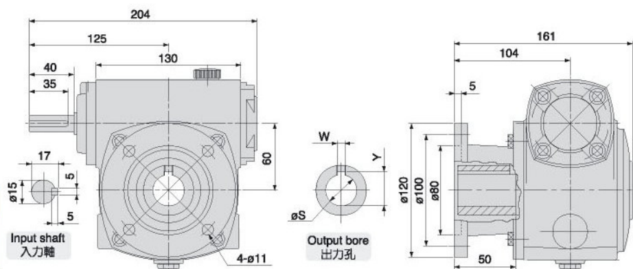
尺寸表 Dimension(m/m)
