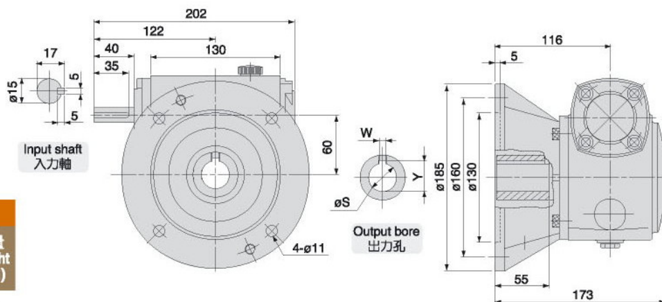
尺寸表 Dimension(m/m)
