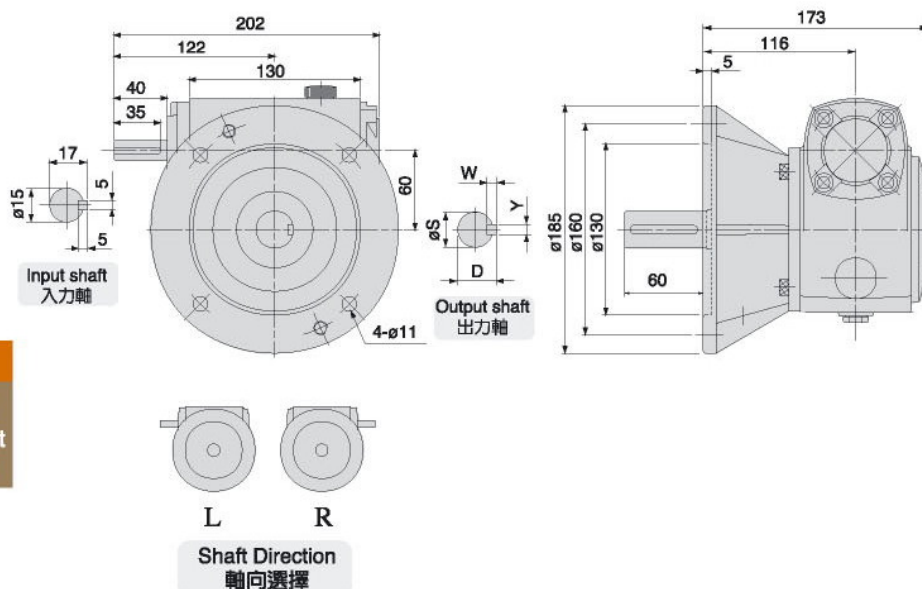
尺寸表 Dimension(m/m)
