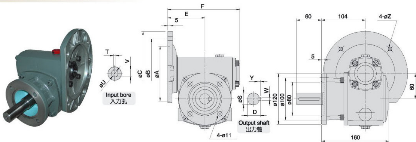
尺寸表 Dimension
