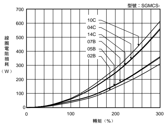
(f) DD馬達 SGMCS 型
