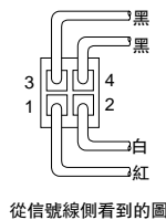
從信號線側看到的圖
