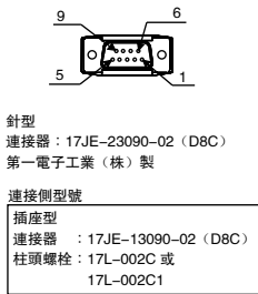
霍爾位置檢知器用連接器規格
