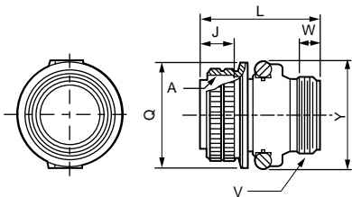
(a) MS3106B：直插頭分體式外殼的外形圖
