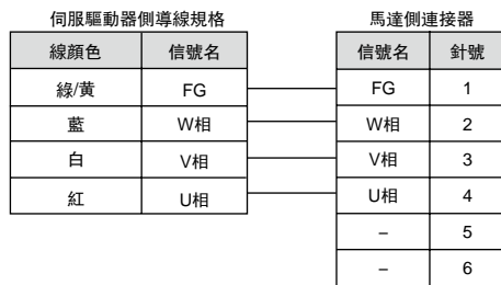
(1) 不帶保持煞車器的伺服馬達接線規格: 100 ~ 400W
