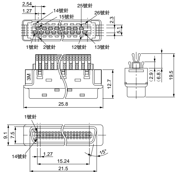
· 連接器外形圖 (單位: mm)
