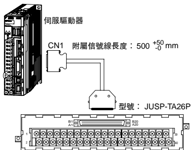
· 附屬信號線外形圖 (單位: mm)
