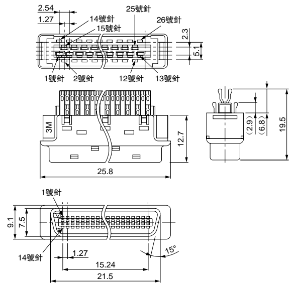
· 連接器外形圖 (單位: mm)
