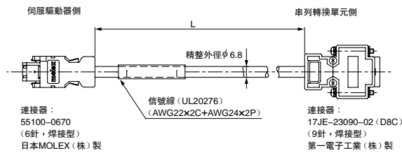
(3) 串列轉換單元連接信號線 (JZSP-CLP70-□□-E 型)
