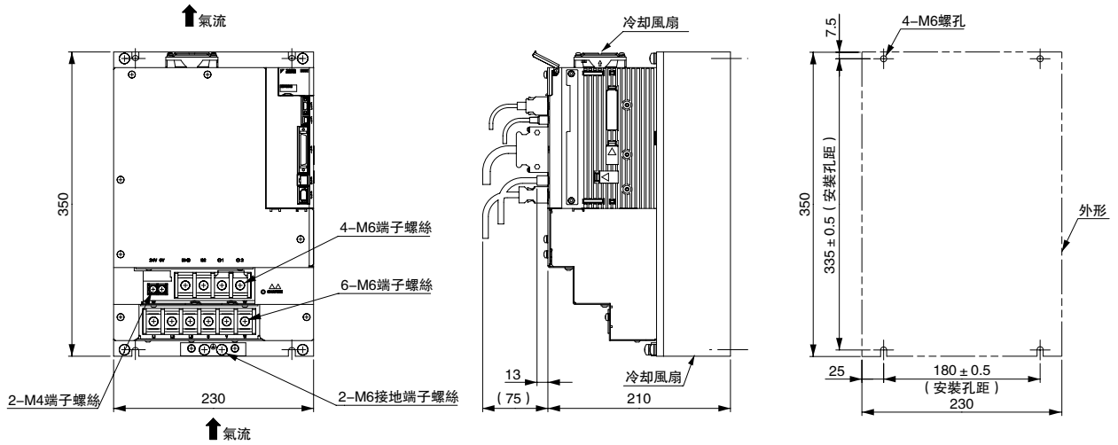
安裝孔加工圖
