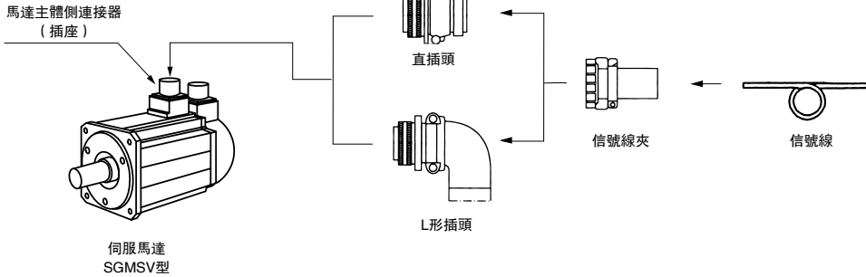
馬達側連接器 1.0 ~ 7.0kW
