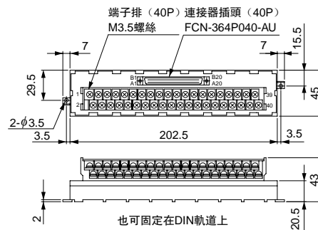
· 端子台外形圖 (單位: mm)
