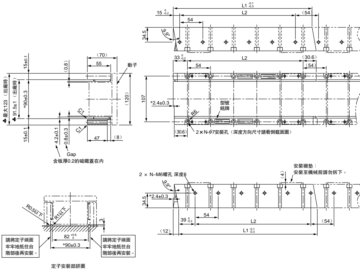
定子安裝部詳圖
