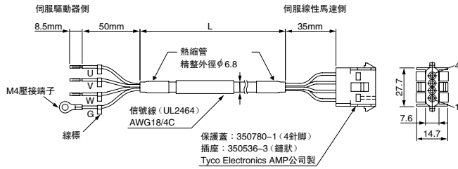
(1) 伺服線性馬達主回路信號線 (JZSP-CLN11-□□-E 型)
