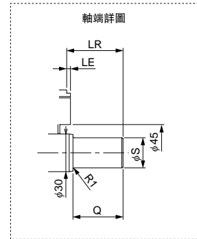
選配軸端規格請參照P.77。
