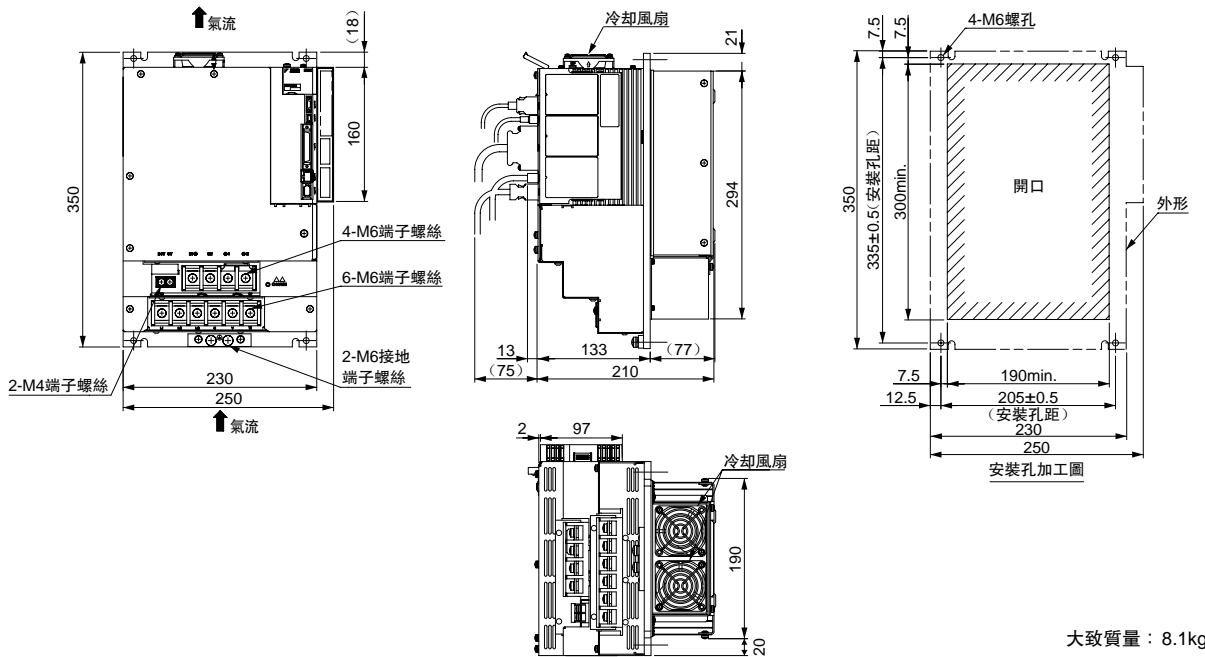
(14) 三相AC400V SGD210D□□A001000□□□, SGD260D□□A001000□□□ (通風管道型)
