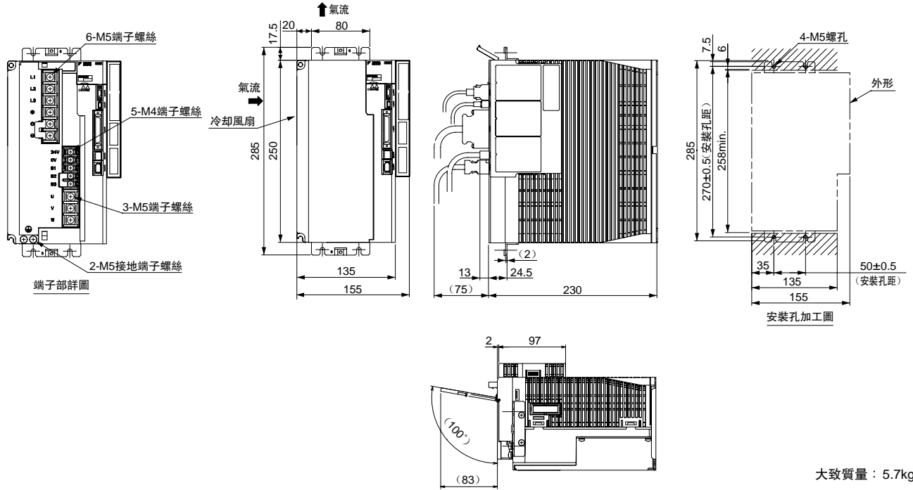
(14) 三相AC400V SGD210D□□A001000□□□, SGD260D□□A001000□□□ (通風管道型)
