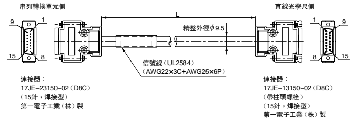
(2) 直線光學尺連接信號線 (JZSP-CLL00-□□-E 型)
