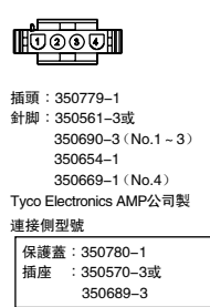
馬達用連接器規格
