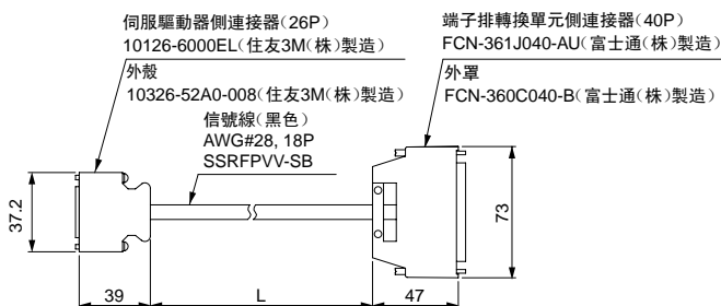
· 附屬信號線外形圖 (單位: mm)
