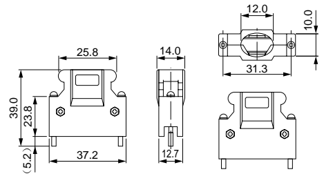
· 外殼外形圖 (單位: mm)
