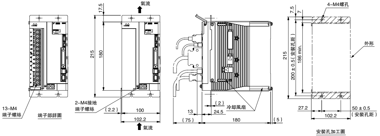
(8) 三相 AC 200V SGD V-330A□□A001
