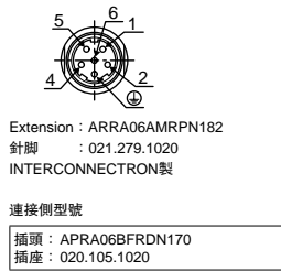
馬達用連接器規格
