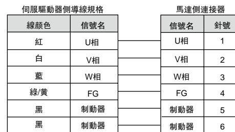
(4) 帶保持煞車器的伺服馬達接線規格: 750W, 1.5kW
