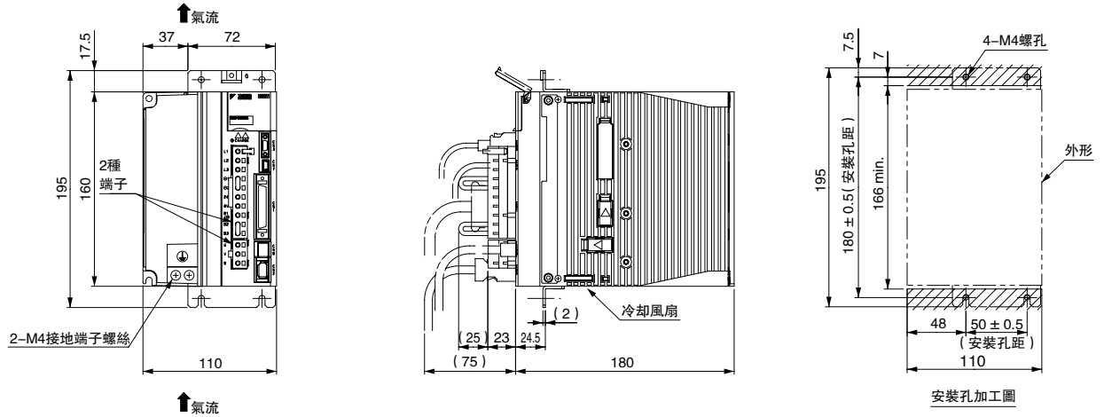
(12) 三相 AC 400V SGDV-8R4D□□A001, -120D□□A001
