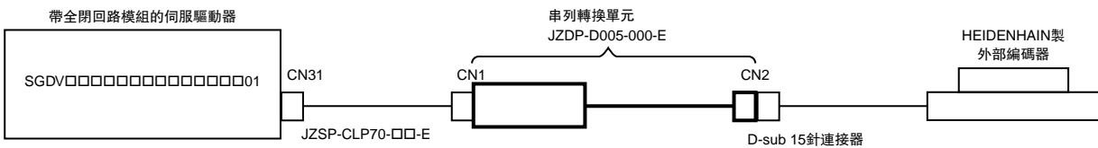
CN1
