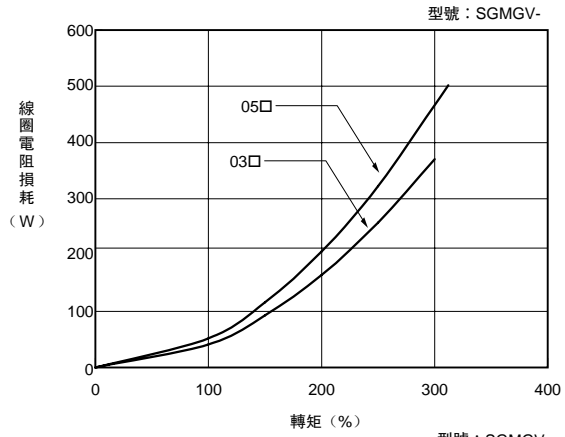
(d) 旋轉型伺服馬達 SGMGV 型
