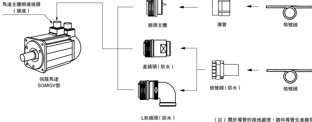
馬達側連接器 0.85 ~ 15kW
